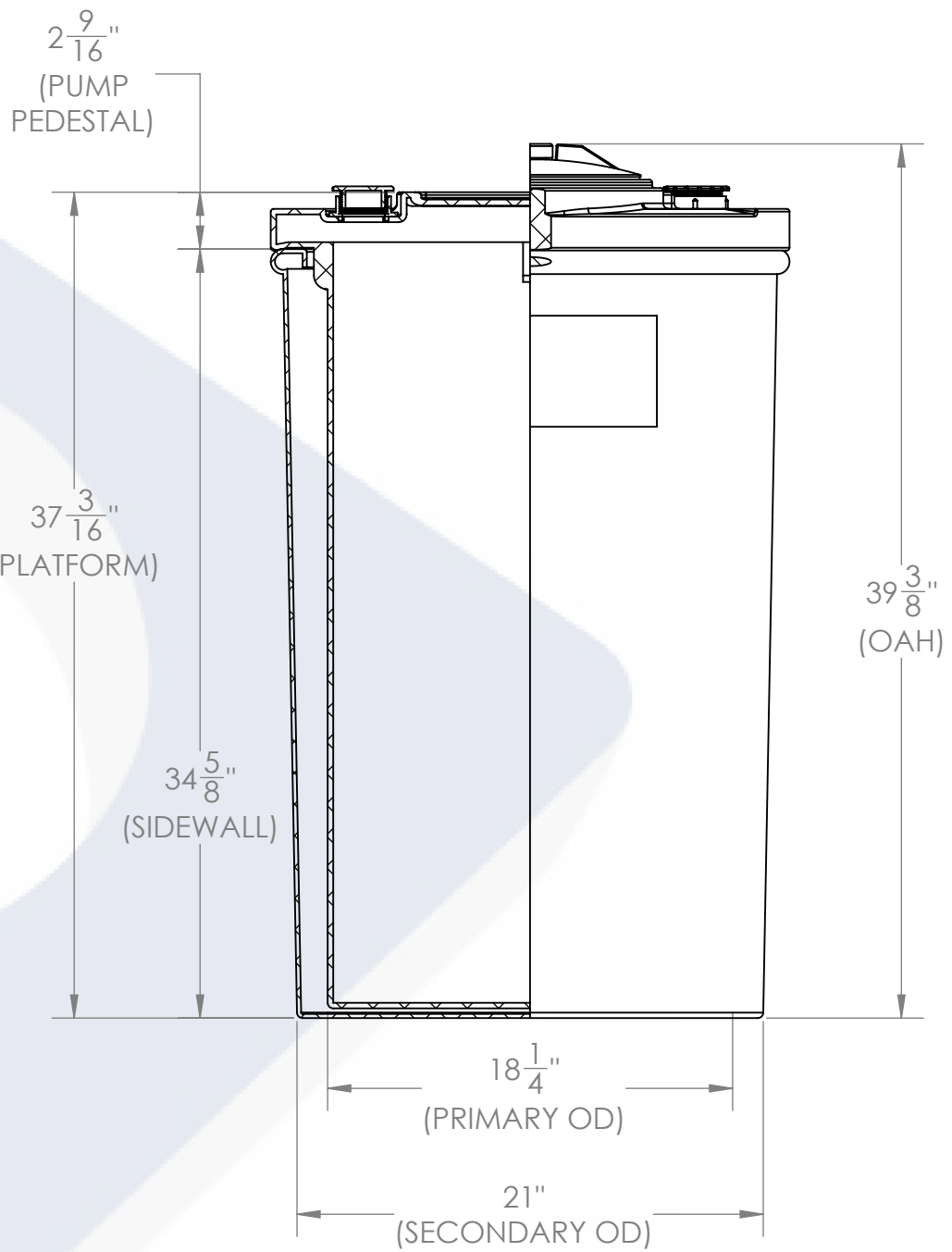
SECTION A-A
